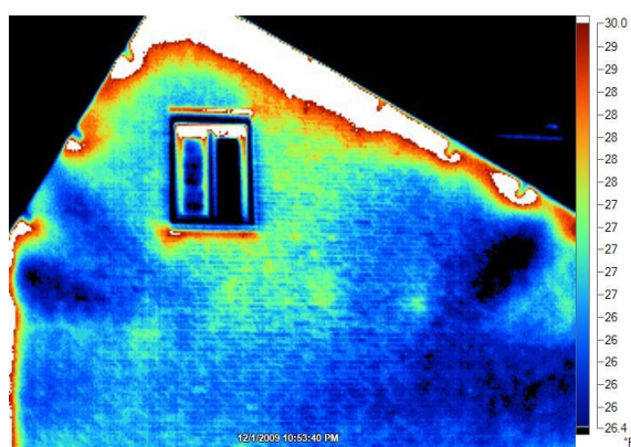
figuur 5.2 Infrarood foto van een zijgevel met warmtelekken
